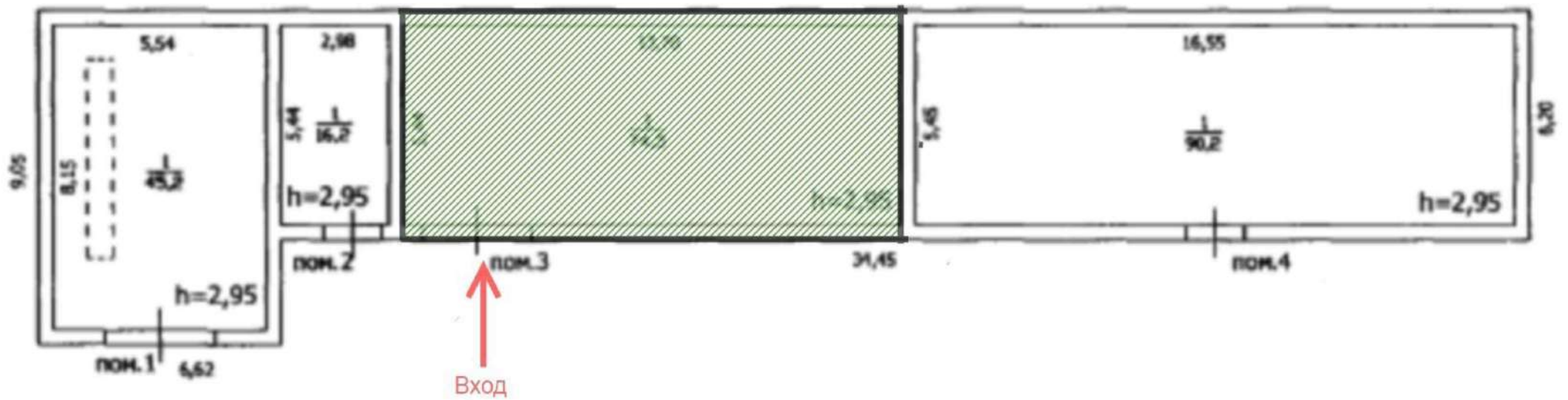
План склада-гаража 74,5 кв.м. ул. Пограничников, 35
