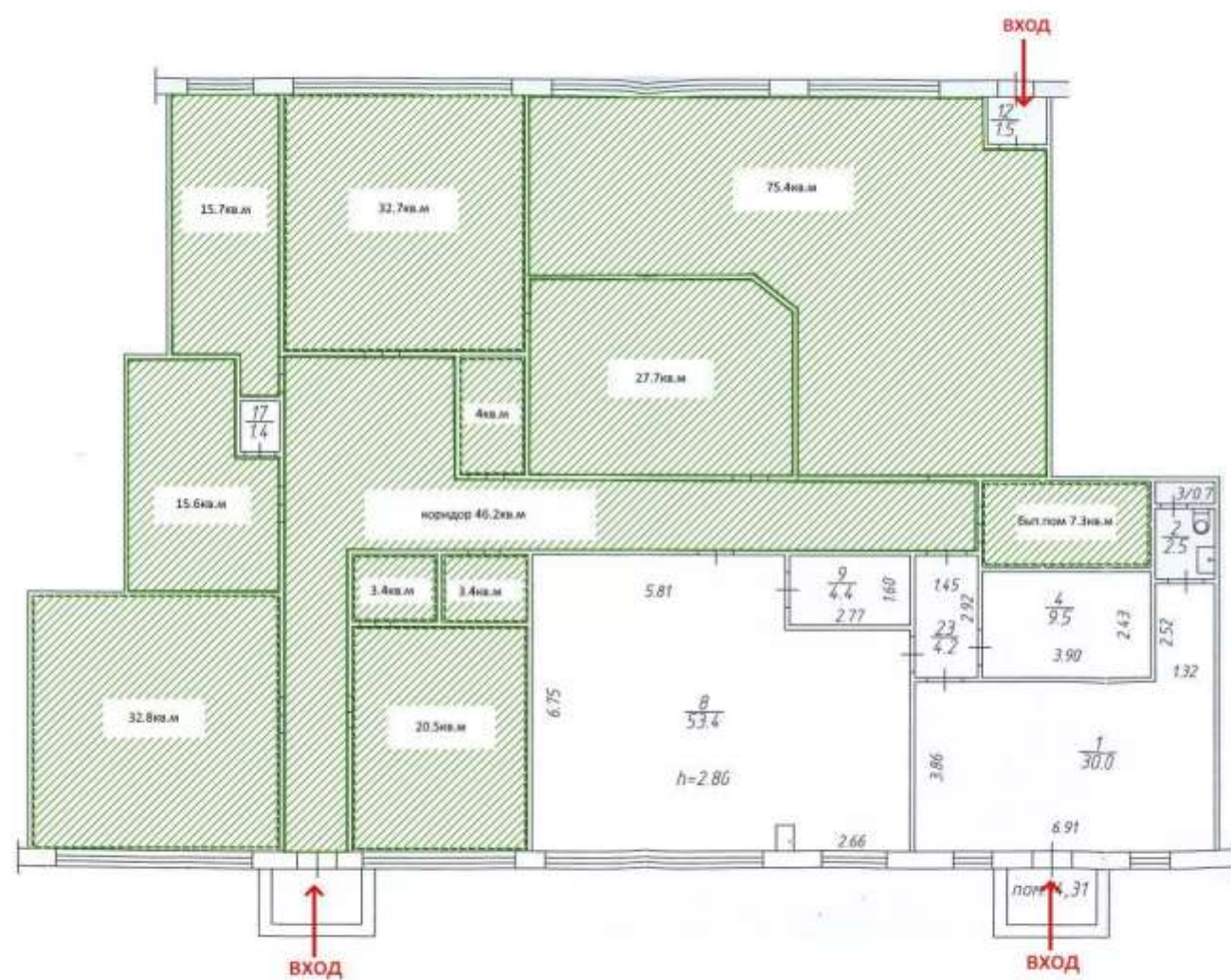
План 1 этажа
